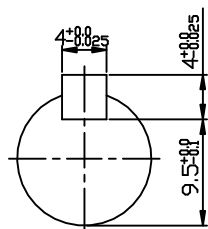
INPUT SHAFT
