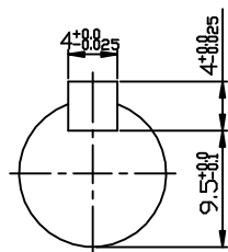
INPUT SHAFT
