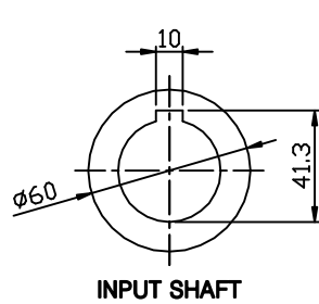
INPUT SHAFT
