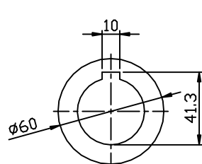
INPUT SHAFT
