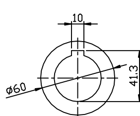
INPUT SHAFT
