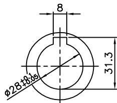
INPUT SHAFT
