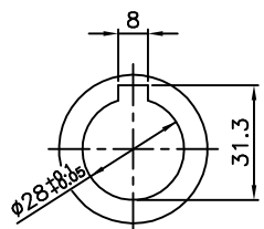
INPUT SHAFT
