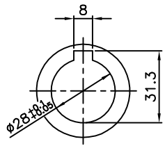
INPUT SHAFT
