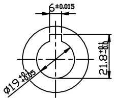
INPUT SHAFT
