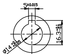
INPUT SHAFT
