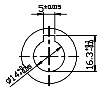
INPUT SHAFT
