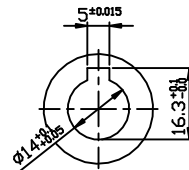
INPUT SHAFT
