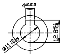
INPUT SHAFT
