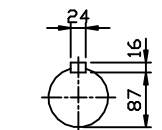
INPUT SHAFT
