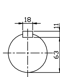
INPUT SHAFT
