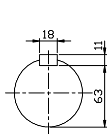
INPUT SHAFT
