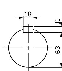
INPUT SHAFT
