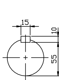
INPUT SHAFT
