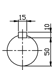
INPUT SHAFT
