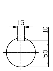
INPUT SHAFT
