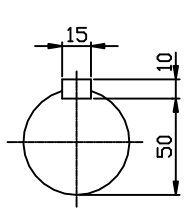
INPUT SHAFT
