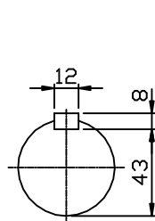
INPUT SHAFT
