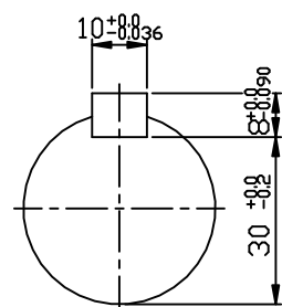
INPUT SHAFT
