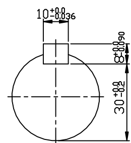
INPUT SHAFT
