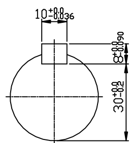
INPUT SHAFT
