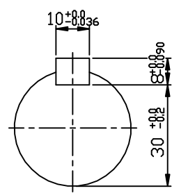
INPUT SHAFT
