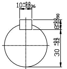
INPUT SHAFT
