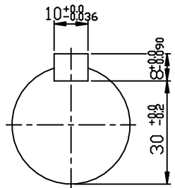
INPUT SHAFT
