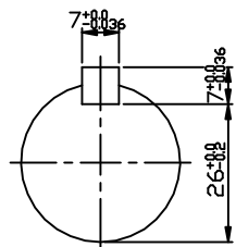
INPUT SHAFT
