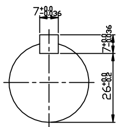
INPUT SHAFT
