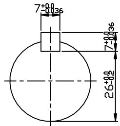
INPUT SHAFT
