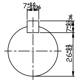
INPUT SHAFT
