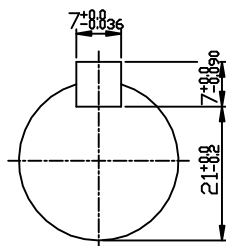
INPUT SHAFT
