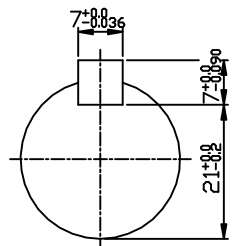
INPUT SHAFT
