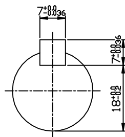
INPUT SHAFT
