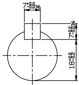
INPUT SHAFT
