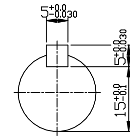
INPUT SHAFT
