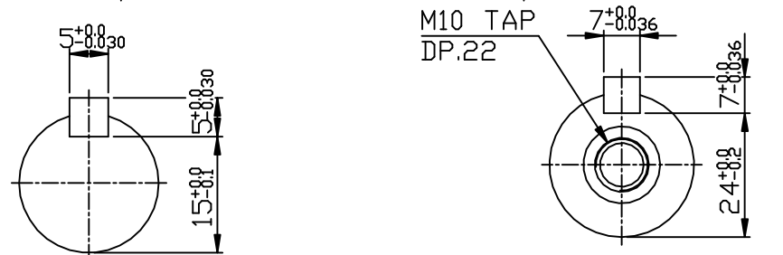
INPUT SHAFT
