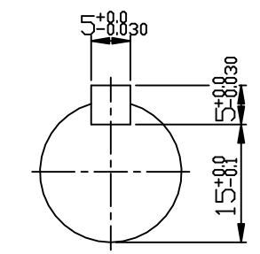
INPUT SHAFT
