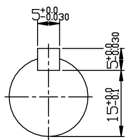
INPUT SHAFT
