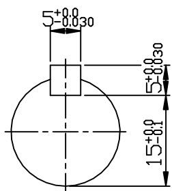
INPUT SHAFT
