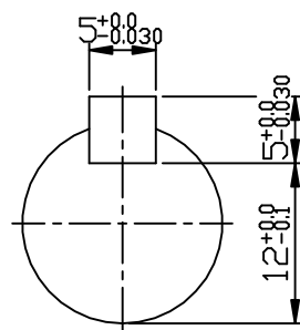
INPUT SHAFT
