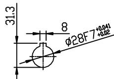
INPUT SHAFT
