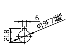
INPUT SHAFT
