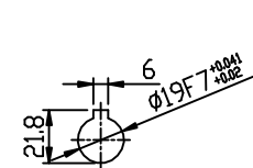
INPUT SHAFT
