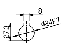
INPUT SHAFT
