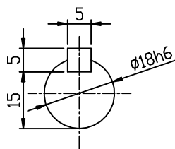
INPUT SHAFT
