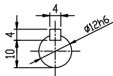
INPUT SHAFT
