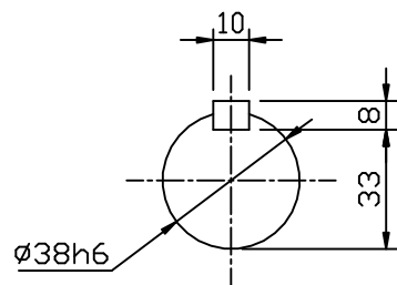
INPUT SHAFT
