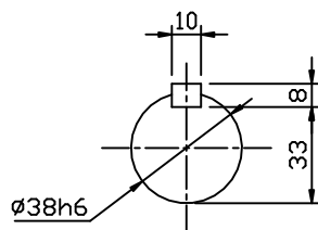
INPUT SHAFT
